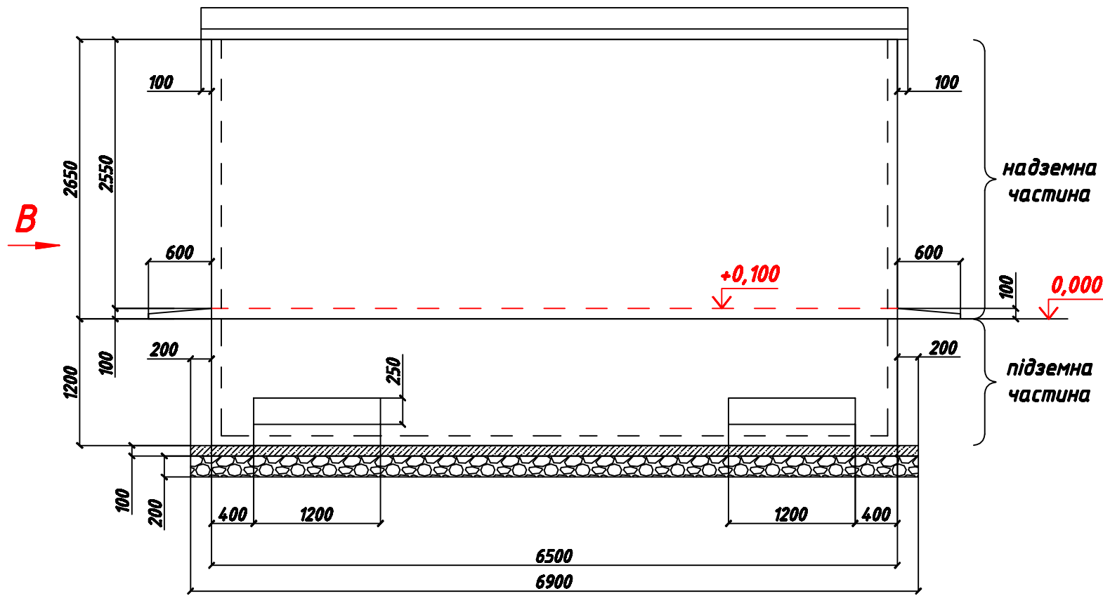
Вид Б
