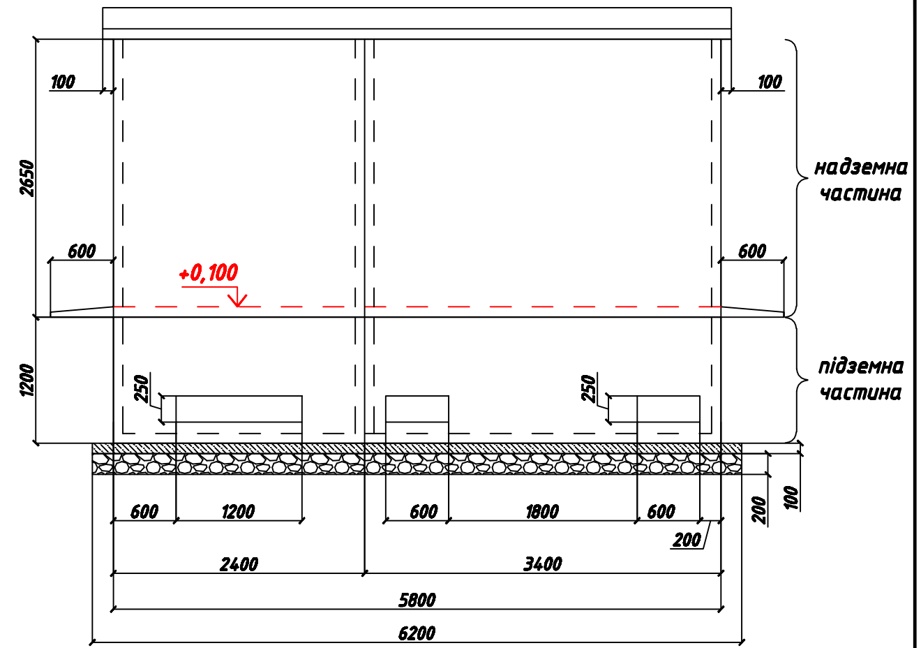
Вид В
